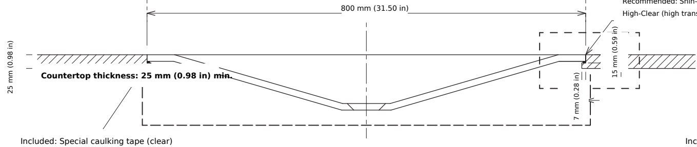
A-A' Section
