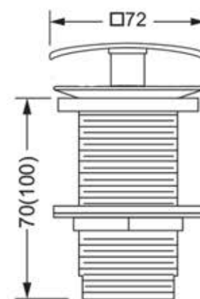
JORGER排水栓本体図
