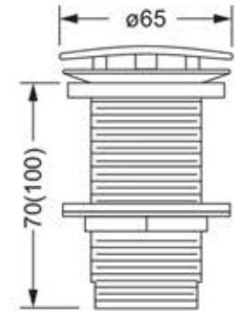
JORGER排水栓本体図
